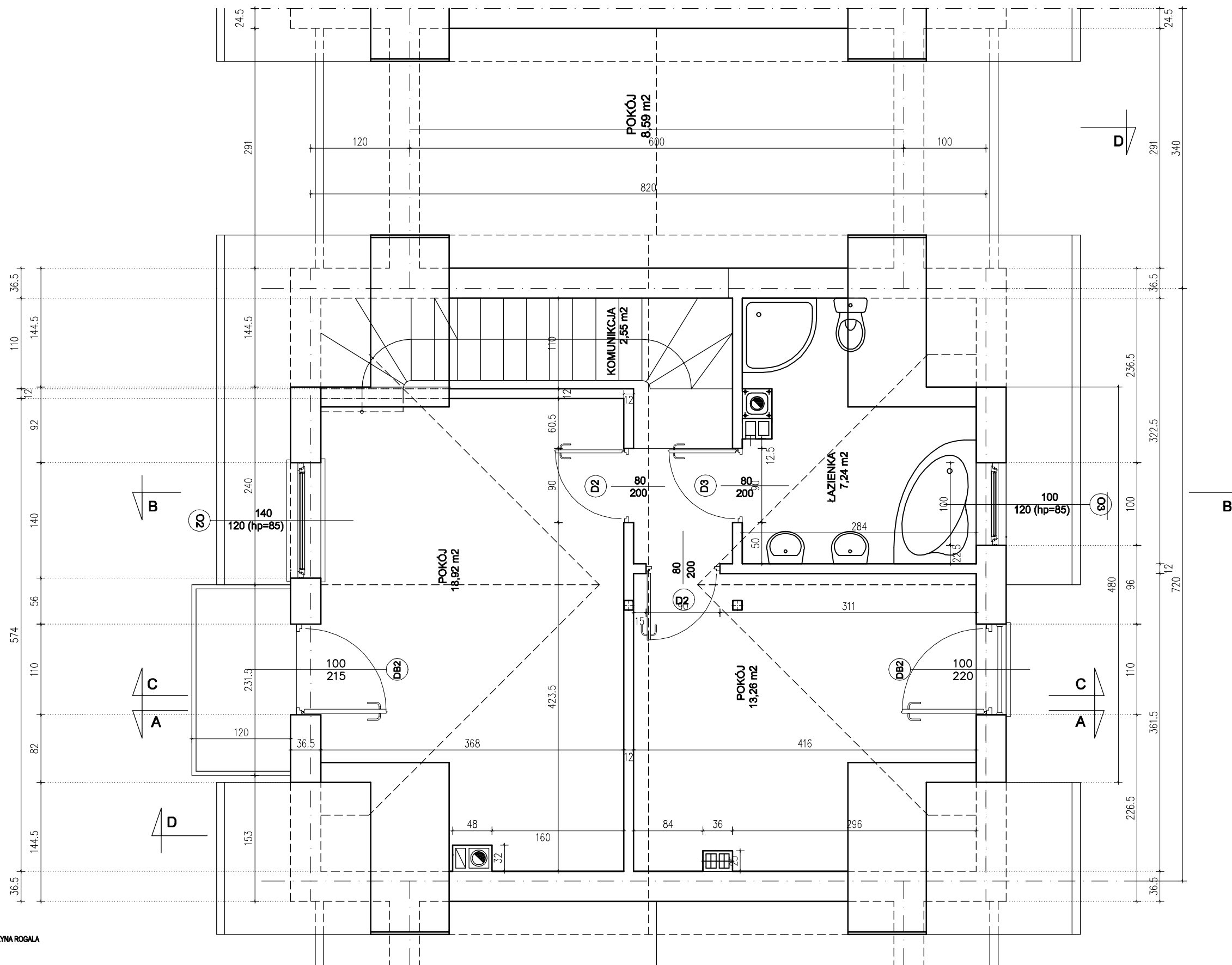
RZUT PODDASZA 41,97 m 2 p.u.
